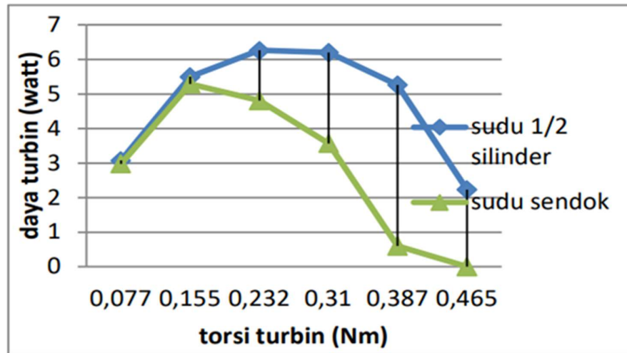
Gambar 1. Grafik Hubungan Torsi Turbin Terhadap Daya Turbin Katup Bukaan Penuh (Full Opened Valve). Sumber: (Madagaskar, 2022)
